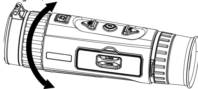
Abbildung 3-2 Fokus einstellen
