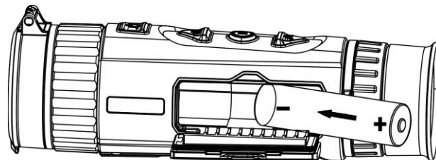
Abbildung 2-4 Akku einsetzen
